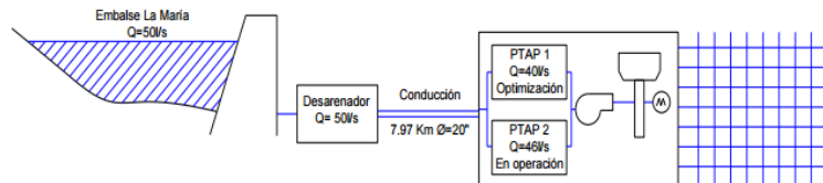
Ilustración 1 Esquema estructural servicio de acueducto
